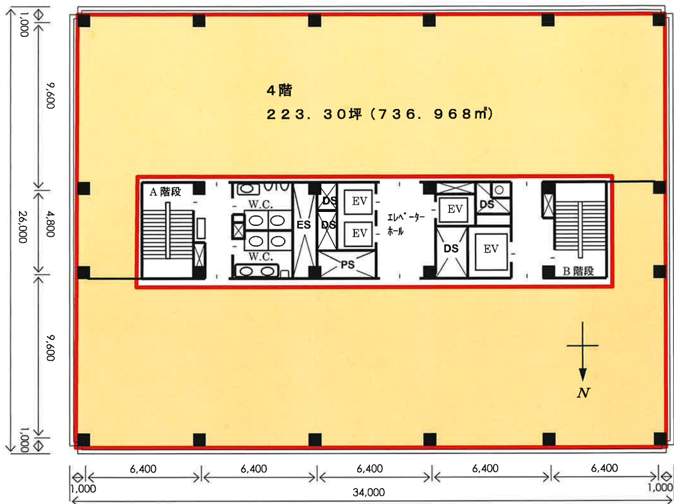
龍名館本店ビル4階平面図
