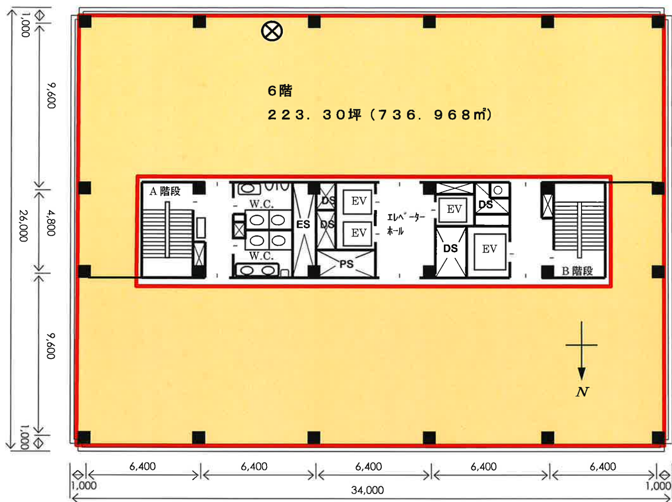
龍名館本店ビル6階平面図
